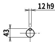
入力軸
