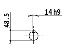
入力軸
