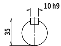
出力軸 (尺度1/2)
