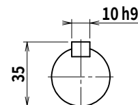
出力軸 (尺度1/2)
