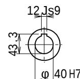
中空出力軸 (尺度 1/6)
