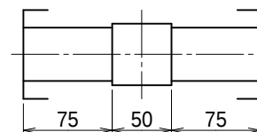
出力軸内部詳細 (尺度1/4)
