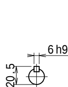
入力軸 (尺度1/3)
