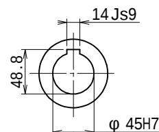
出力軸 (尺度1/4)
