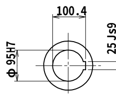
出力軸
