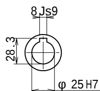
出力軸 (尺度 1/3)
