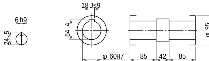
出力軸内部詳細 (尺度 1/5)
