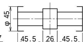
出力軸内部詳細 (尺度 1/3)
