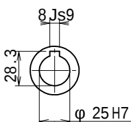
出力軸 (尺度 1/3)
