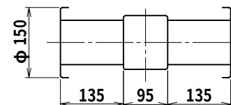
出力軸内部詳細
