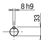
入力軸
