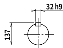
出力軸
