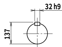
出力軸
