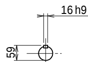
入力軸
