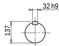
出力軸
