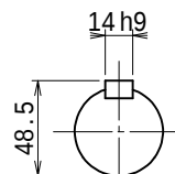
出力軸 (尺度 1/3)
