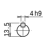
入力軸 (尺度1/1.5)
