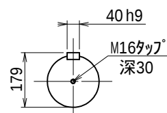
出力軸 (S=1/12)
