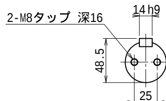
出力軸
