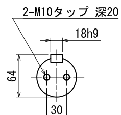
出力軸 (尺度1/4)
