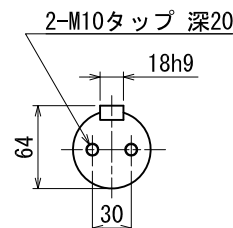
出力軸 (尺度1/4)
