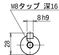
出力軸 (尺度 1/2)
