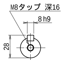
出力軸 (尺度 1/2)
