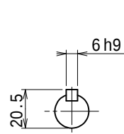
入力軸 (尺度 1/2)
