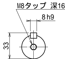
出力軸 (尺度 1/2)
