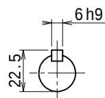
入力軸 (尺度 1/2)
