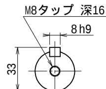
出力軸 (尺度 1/2)
