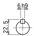
入力軸 (尺度 1/2)
