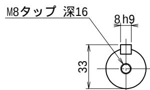
出力軸 (尺度 1/2)
