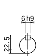
入力軸 (尺度 1/2)
