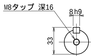
出力軸 (尺度 1/2)
