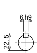
入力軸 （尺度 1/2）
