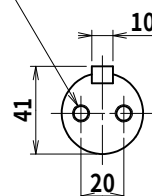
出力軸 (尺度 1/2.5)
