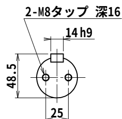
出力軸 (尺度1/3)
