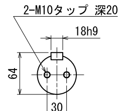
出力軸 (尺度1/4)
