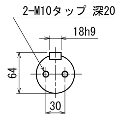
出力軸 (尺度1/4)
