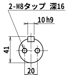
出力軸 (尺度 1/2.5)
