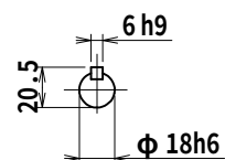
入力軸 (尺度1/3)
