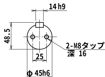
出力軸 (尺度1/3)
