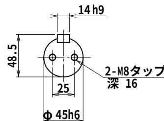
出力軸 (尺度1/3)
