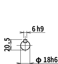
入力軸 (尺度1/3)
