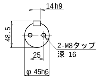
出力軸 (尺度1/3)
