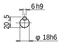
入力軸 (尺度1/3)
