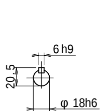
入力軸 (尺度1/3)
