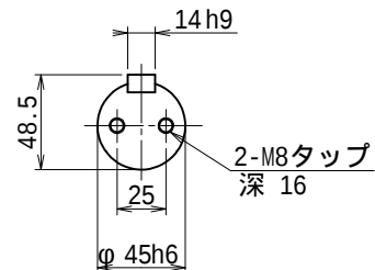
出力軸 (尺度1/3)
