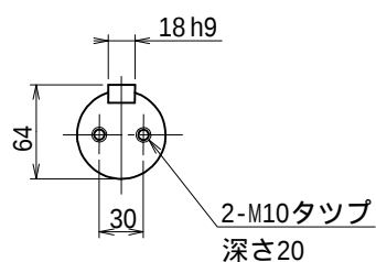
出力軸
