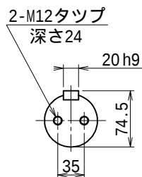
出力軸
