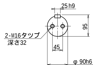
出力軸
