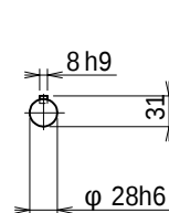
入力軸
