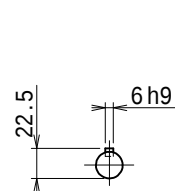
入力軸
