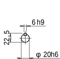
入力軸
