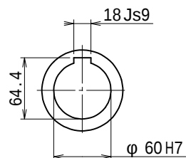
出力軸
