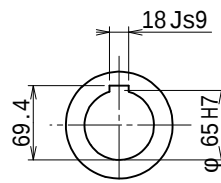
出力軸 (尺度 1/5)
