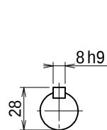
入力軸 (尺度 1/2.5)
