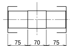
出力軸内部詳細 (尺度 1/5)
