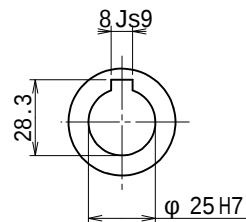
出力軸
