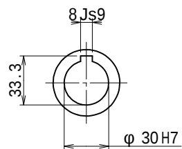
出力軸
