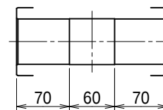
出力軸内部詳細 (尺度1/4)
