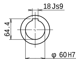
出力軸 (尺度1/4)
