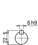
入力軸 (尺度 1/2)
