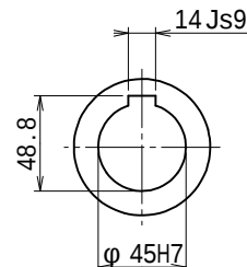
出力軸 (尺度 1/3)
