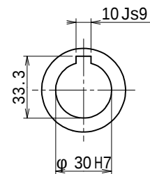
出力軸 (尺度 1/2)
