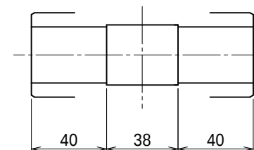
出力軸内部詳細 (尺度 1/2)
