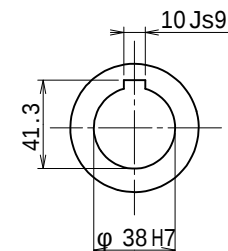
出力軸 (尺度 1/2.5)
