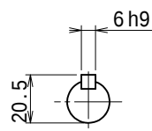
入力軸 (尺度 1/2)
